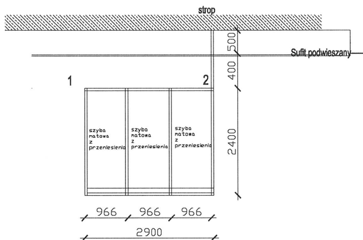
WIDOK 2-3
