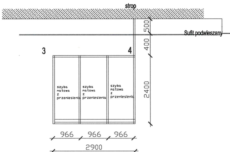
WIDOK 3-4
